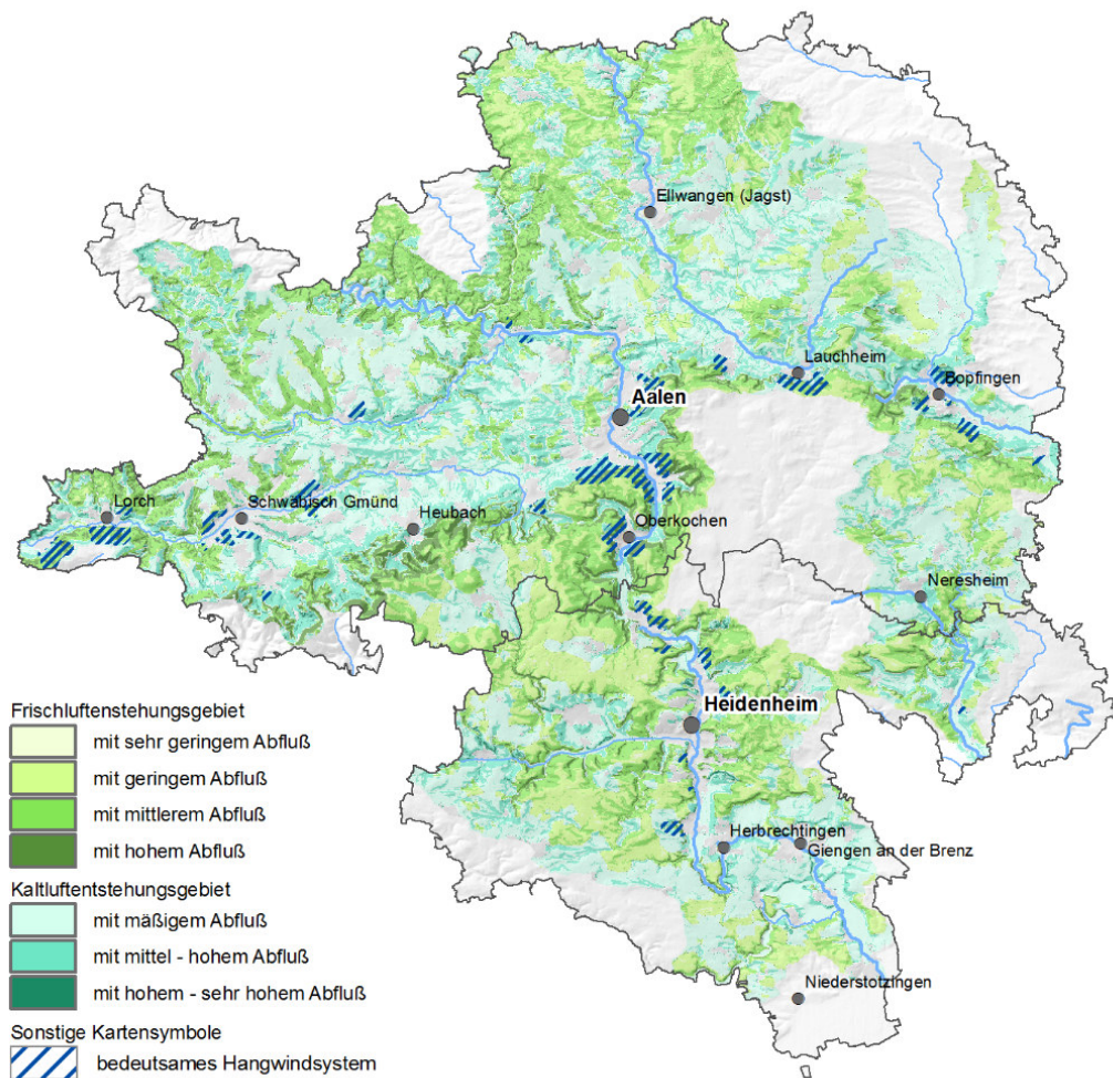
Abbildung 15: Frisch- und Kaltluftentstehungsgebiete im Einzugsgebiet der regional bedeutsamen Luftleitbahnen und bedeutende Hangwindsysteme (RVO 2017)
