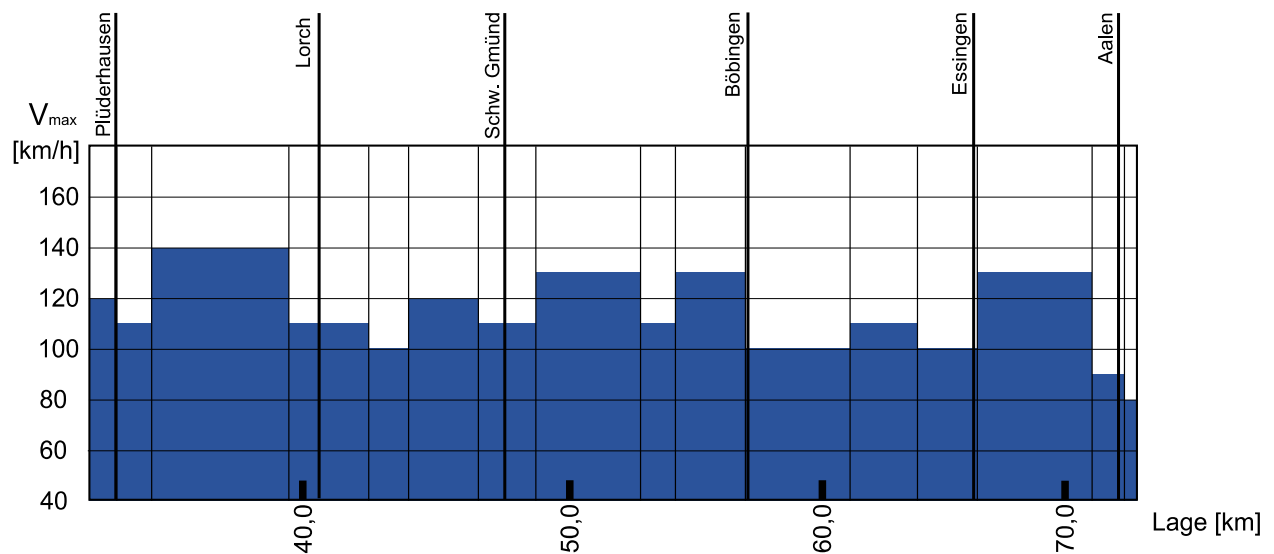
Abbildung 2: Geschwindigkeitsband Remsbahn
